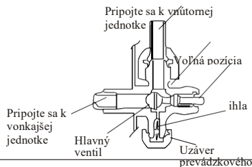
Schéma trojcestného ventilu
