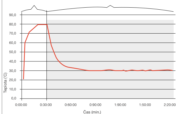
Vývoj povrchové teploty panelu GLOA 2 kW po zapnutí a vypnutí
